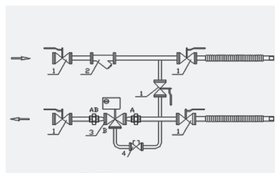
Схема узла терморегулирования Исполнение 2
