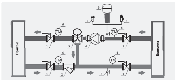
Схема узла терморегулирования для гликолевых рекуператоров SMUT-P
