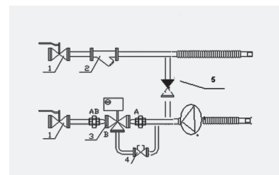
Схема узла терморегулирования Исполнение 3
